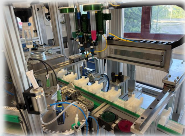
Klebeinheit mit Handling
