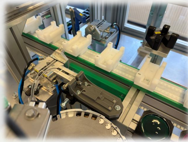
Ausrichtstation und Piezozuführung
